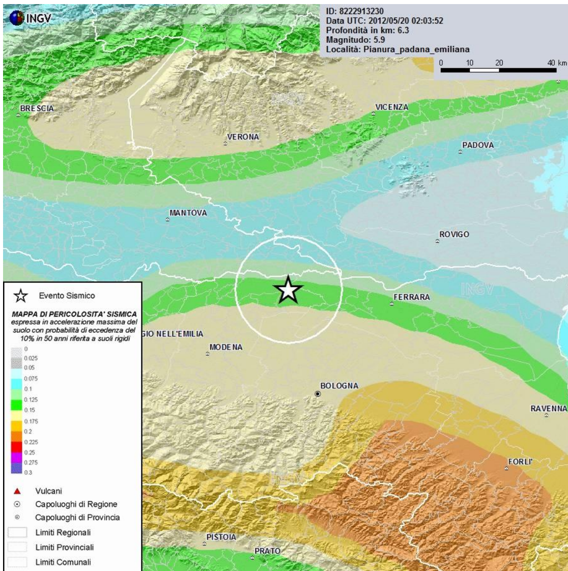
Figura 4. Epicentro del terremoto di MI 5.9 del 20 maggio 2012 e carta di pericolosità sismica nazionale ((GdL MPS, 2004; rif. Ordinanza PCM del 28 aprile 2005, n. 3519, All. 1b) espressa in termini di accelerazione massima del suolo con probabilità di eccedenza del 10% in 50 anni, riferita a suoli rigidi ( V_{s30} > 800 m/s; cat. A, punto 3.2.1 del D.M. 14.09.2005)
